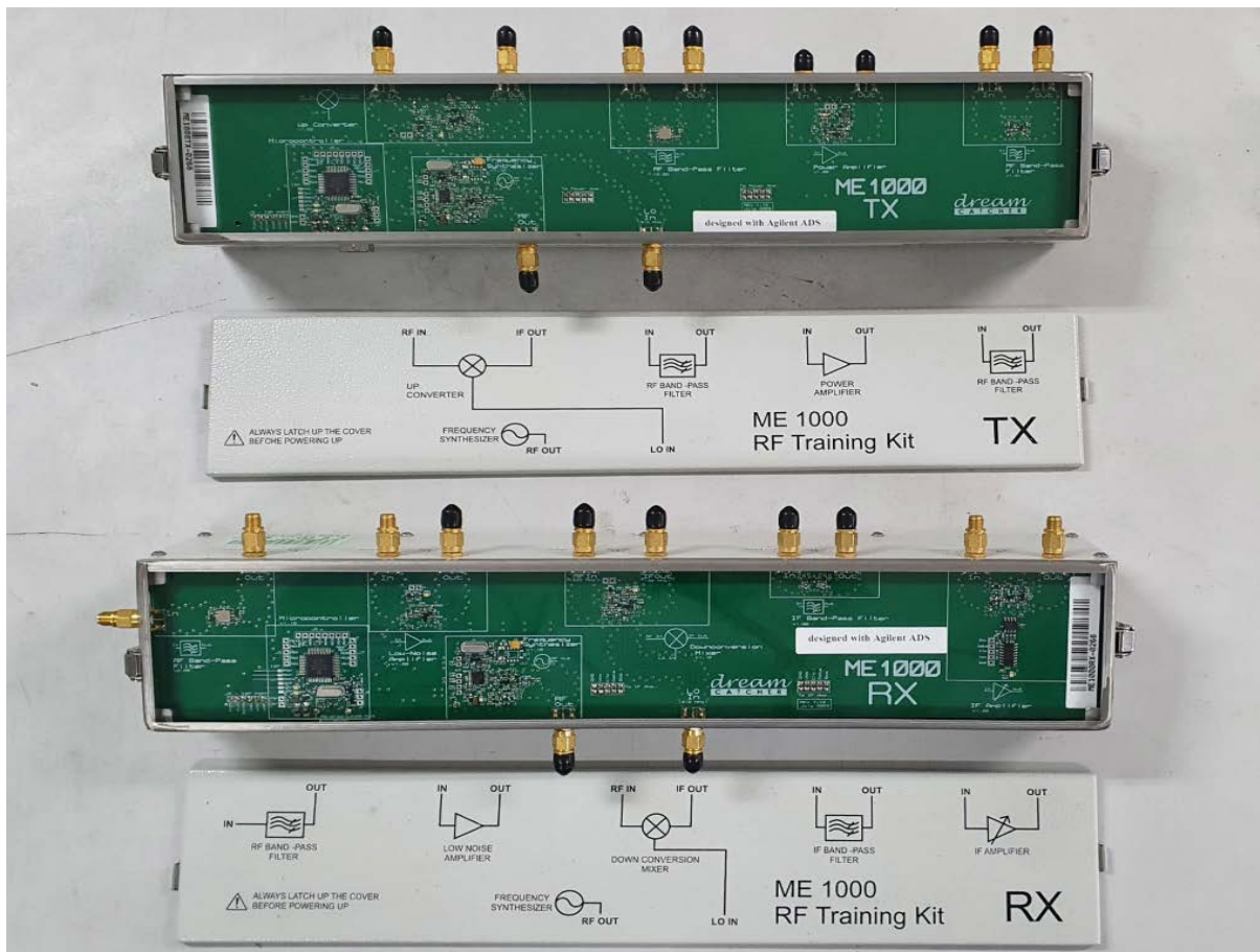
รูปที่ 32 ชุดตรวจวัดอัตราขยายและกรองความถี่สูง
