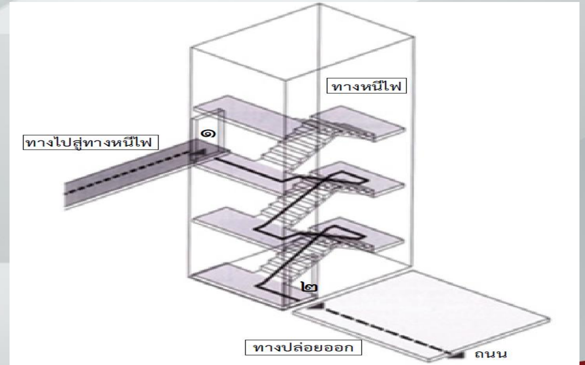
ส่วนประกอบทั้ง 3 ของเส้นทางหนีไฟ ได้แก่ ทาง ไปสู่ทางหนีไฟ (Exit Access) ทางหนีไฟ (Exit) และทางปล่อยออก (Exit Discharge)
