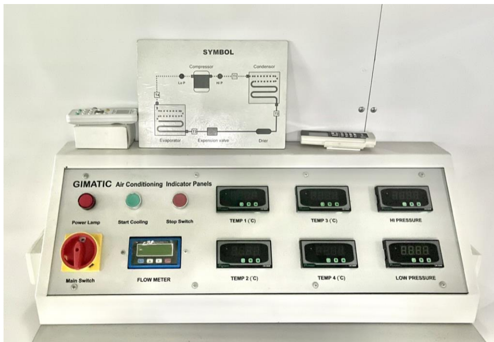
รูปที่ 5.24 ชุดปฏิบัติการการทำความเย็น
