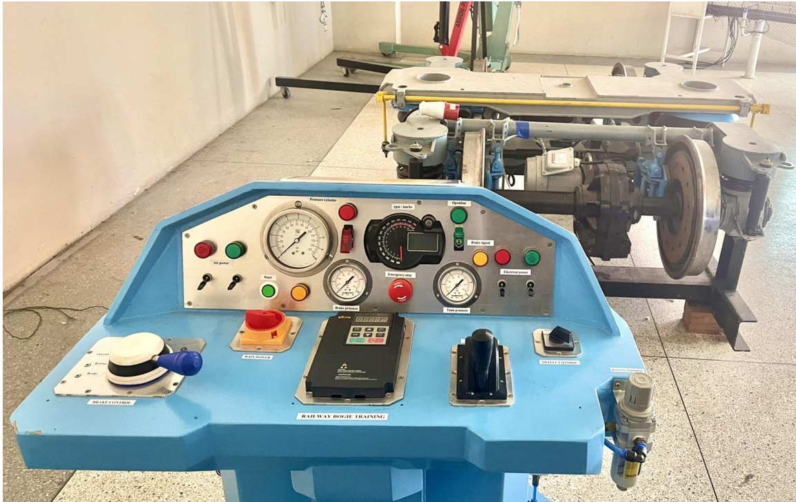
รูปที่ 5.41 ชุดทดสอบระบบเบรกรถไฟ
