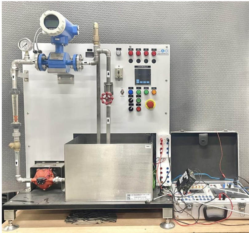
รูปที่ 5.32 ชุดทดลอง Process control
