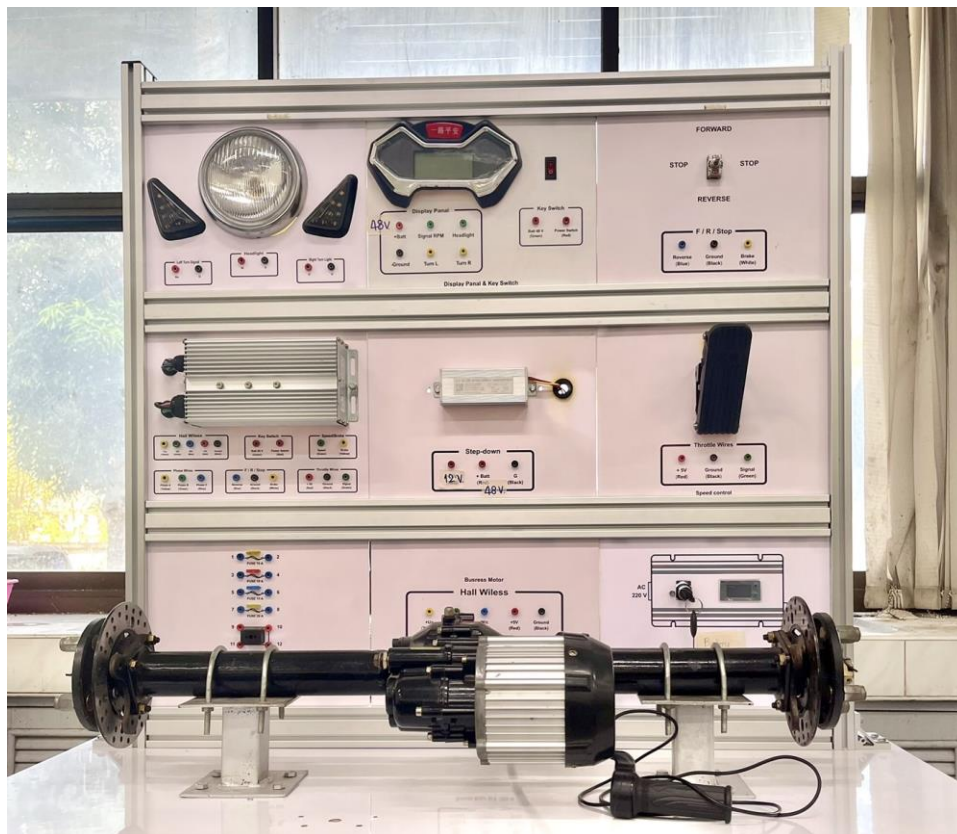
รูปที่ 5.6 ชุดปฏิบัติการยานยนต์ไฟฟ้า (ต่อ)
