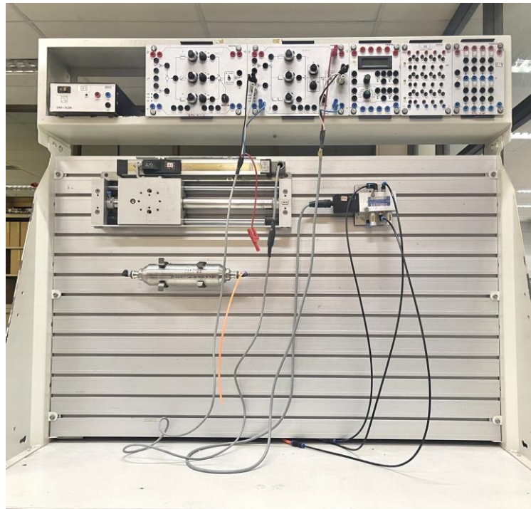
รูปที่ 5.28 ชุดทดลองระบบควบคุมนิวเมติกส์
