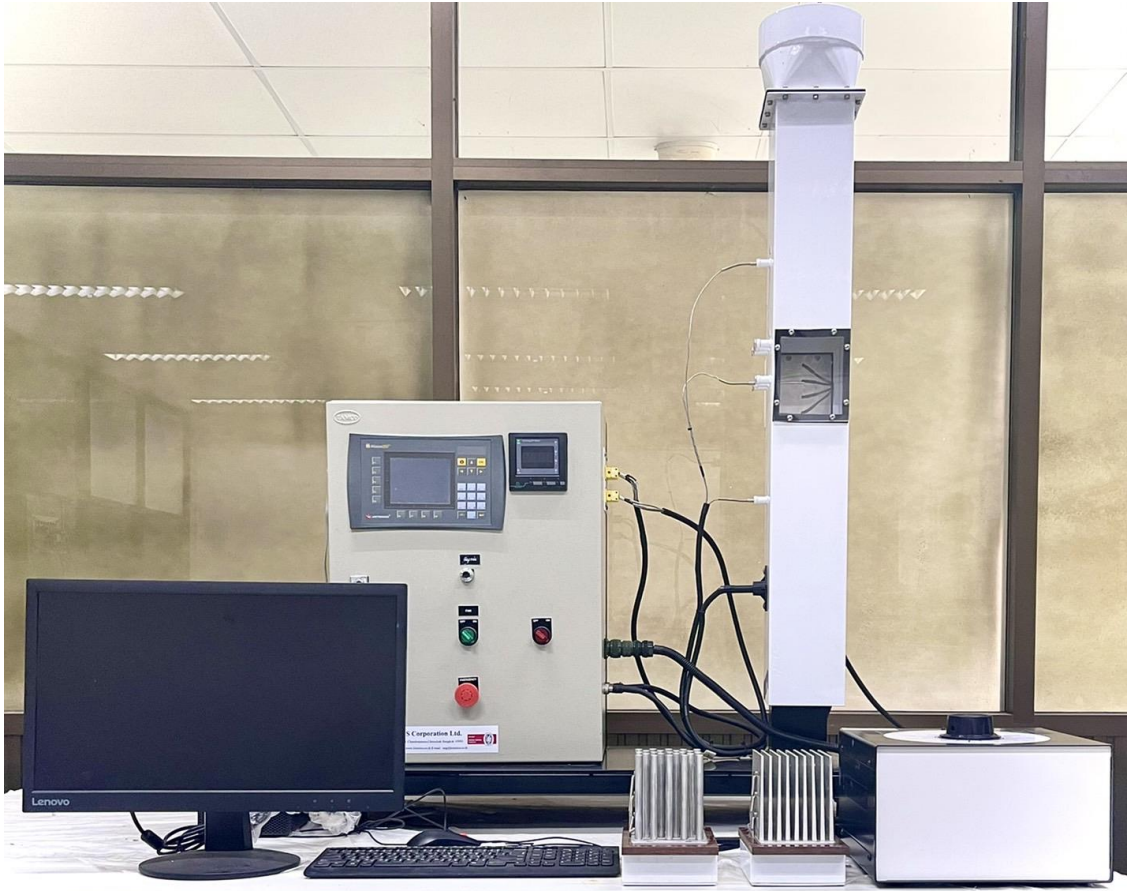
รูปที่ 5.21 ชุดปฏิบัติการทดสอบการระบบการพาความร้อน
