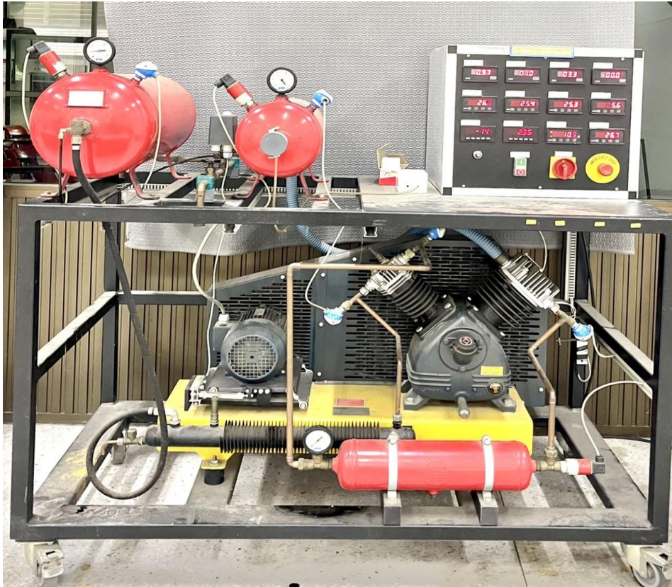
รูปที่ 5.18 ชุดปฏิบัติการเครื่องอัดอากาศ
