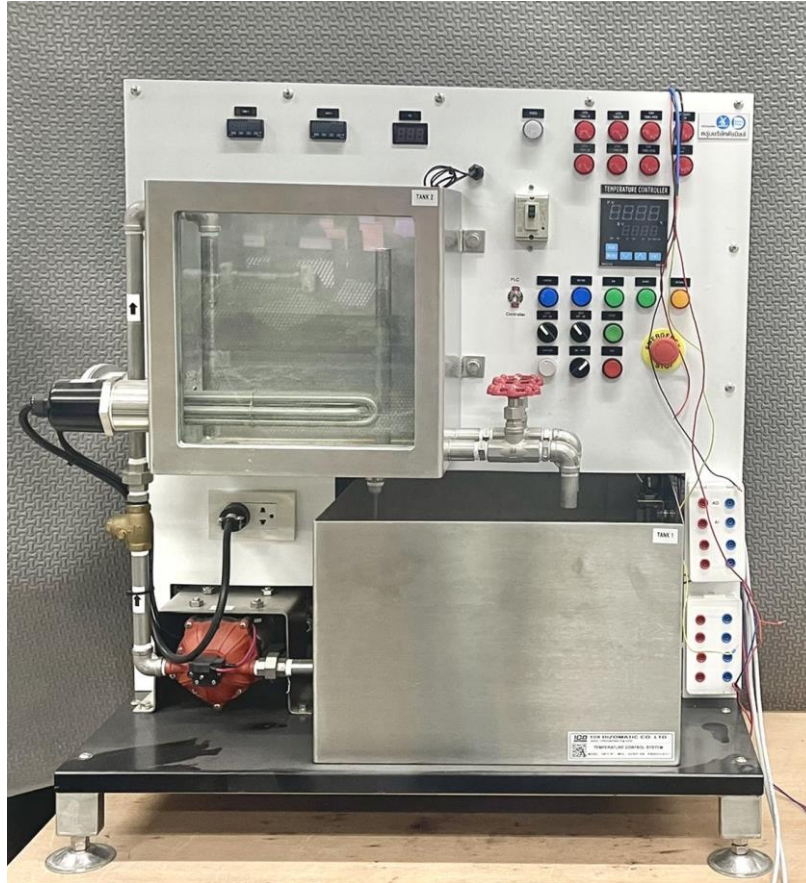
รูปที่ 5.33 ชุดทดลอง Process control
