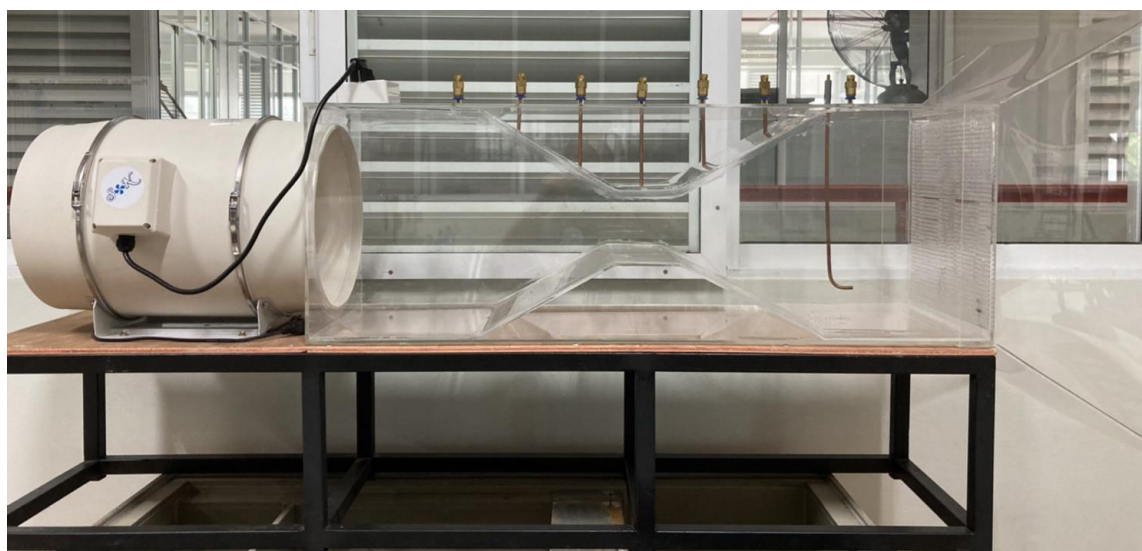
ชุดทดลองการไหลของอากาศ
