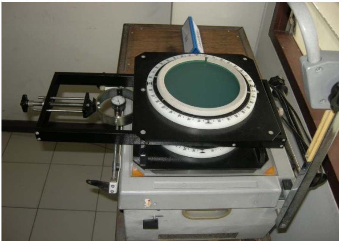
ชุดทดลอง Photo Elastic Polariscopes
