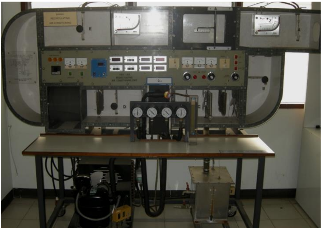
ชุดทดลอง Recirculating Air Conditioning
