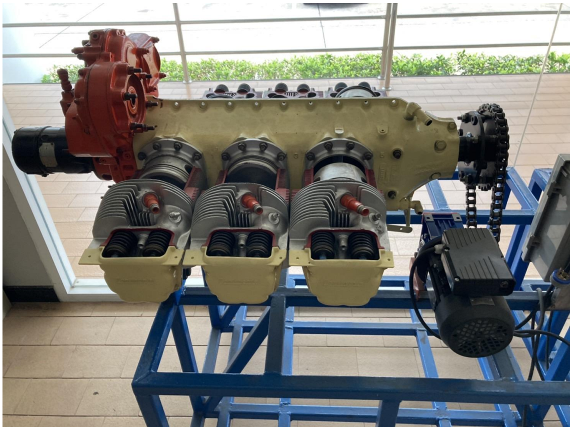
ชุดผ่าเครื่องยนต์ลูกสูบเครื่องบินเล็ก
