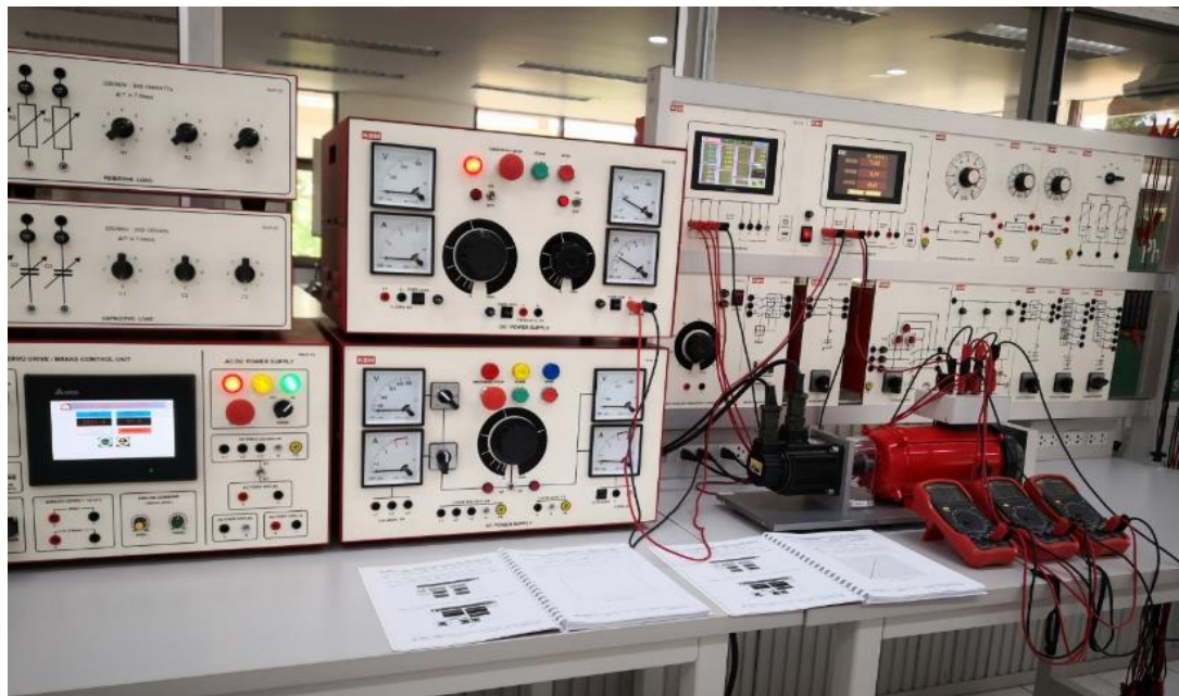
รูปที่ 4.23 ชุดทดลองเครื่องกำเนิดไฟฟ้าซิงโครนัส
