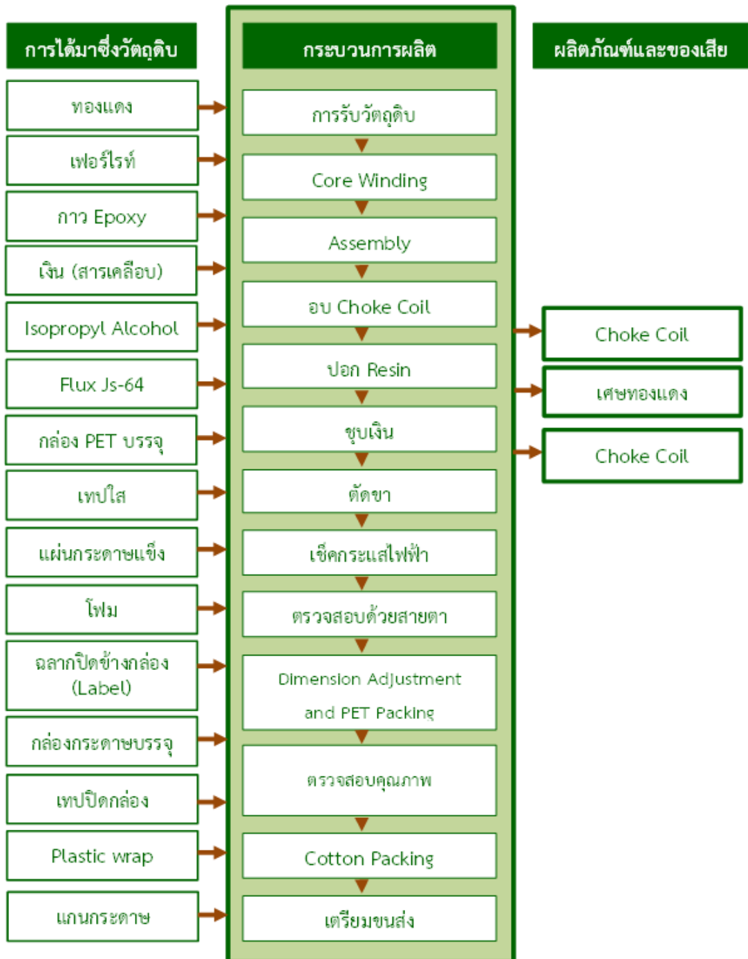
Process Flow Diagram สำหรับการประเมินแบบ B2B
